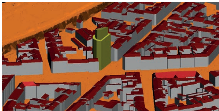
Ryc. 21. Trójwymiarowe modele budynków wykonane na podstawie danych LiDAR. Kolorem żółtym – budynek projektowany
