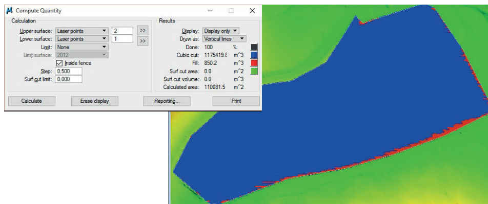
Ryc. 8. Obliczenie objętości wykonane w oprogramowaniu TerraModeler. Na niebiesko – przerost, na czerwono – spadek objętości
