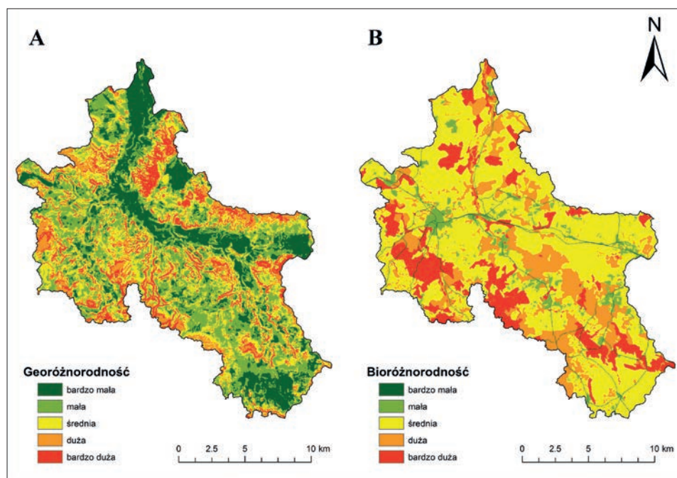
Ryc. 1. Mapy waloryzacji zlewni Dębicy: A – georóżnorodności, B – bioróżnorodności
