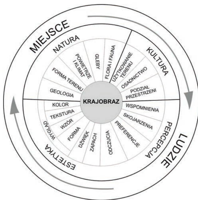
Ryc. 2. Idea krajobrazu w metodzie LCA (Raszeja 2013, za: Swanwick 2002)
