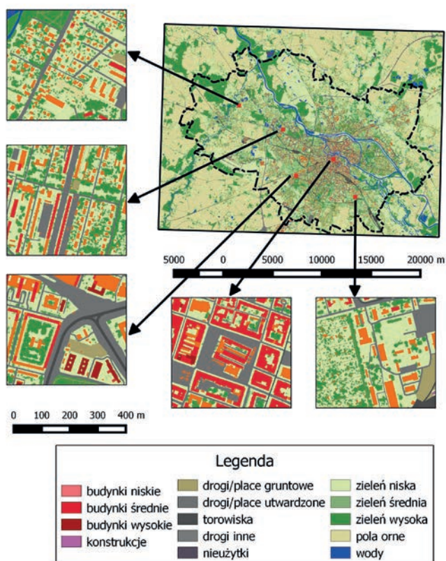
Ryc. 2. Przykładowe fragmenty Szczegółowej Mapy Pokrycia Terenu Wrocławia w układzie geodezyjnym PUG1992
